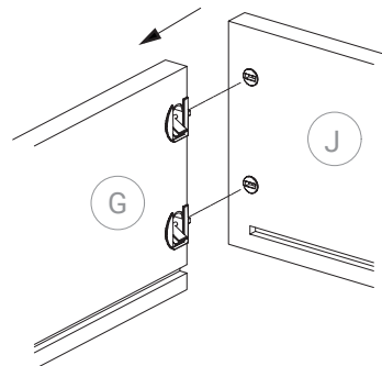
Detalle de la unión / Joint detail
